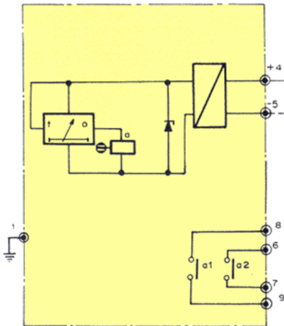
TTT7111 - Schéma de fonctionnement simplifié et de raccordement Simplified operating and connection diagram
